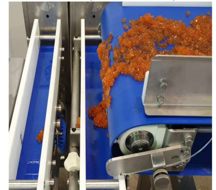
Ejemplo dosificando a 2 puntos ( LMB02)
